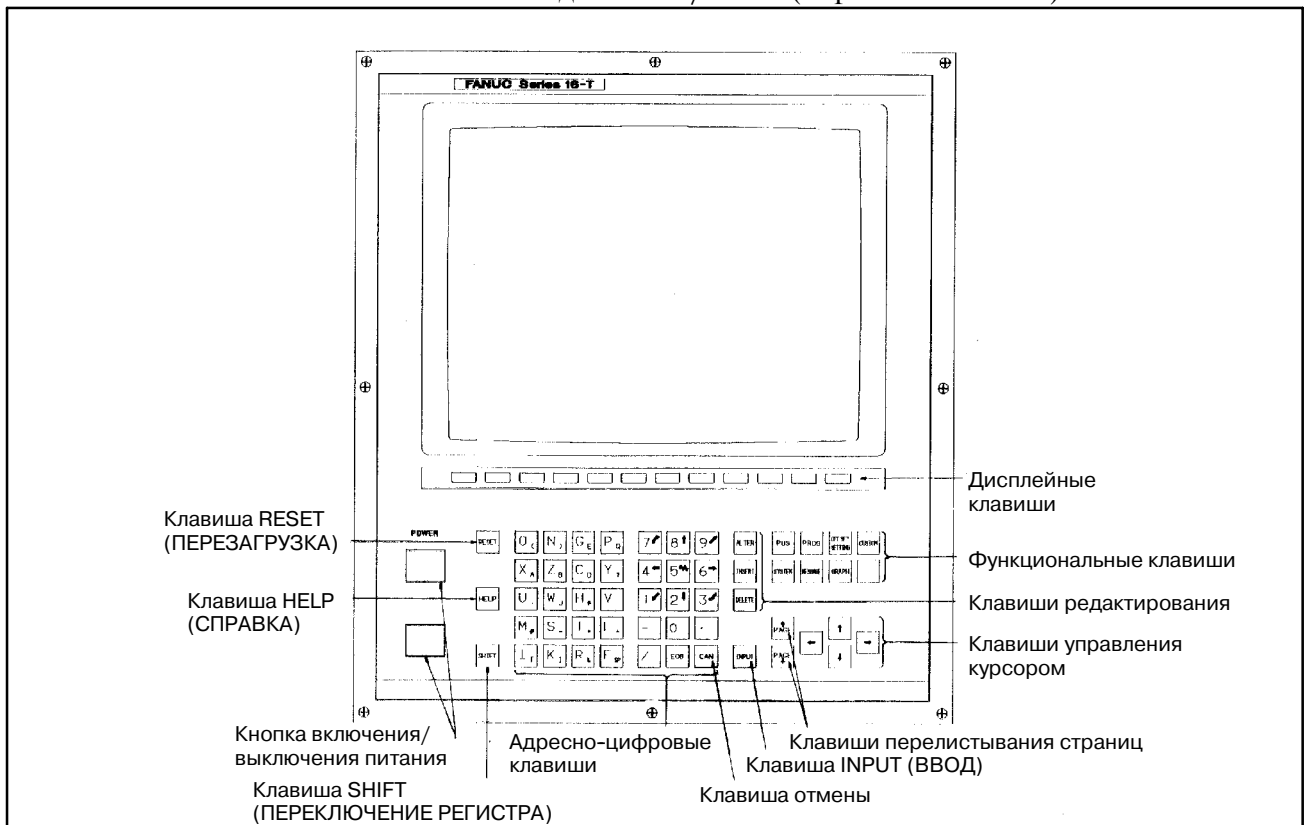
ф) 14" цветной ЭЛТ-монитор/панель ручного ввода данных для 16-ТА/18-ТА (Вертикальный тип)
