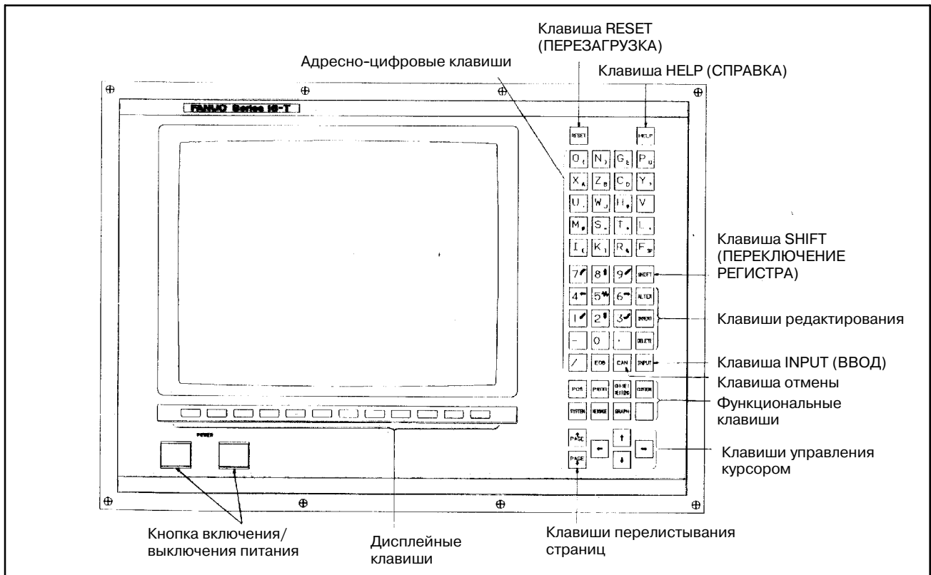
е) 14" цветной ЭЛТ-монитор/панель ручного ввода данных для 16-ТА/18-ТА (Горизонтальный тип)
