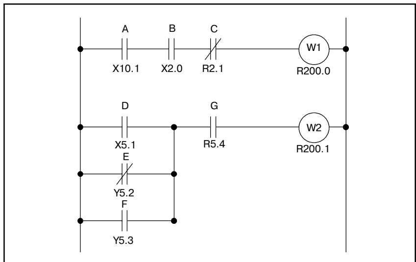
Рис . 4.1.1 Цепная схема
